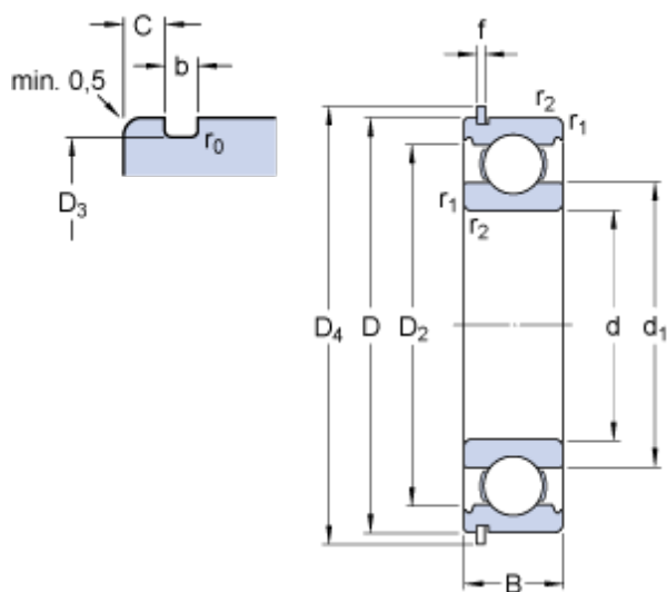
Bearing No. 6303 NR
